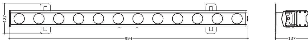
Disegno tecnico
