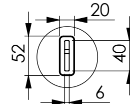
DETAIL A MAßSTAB 1 : 5
